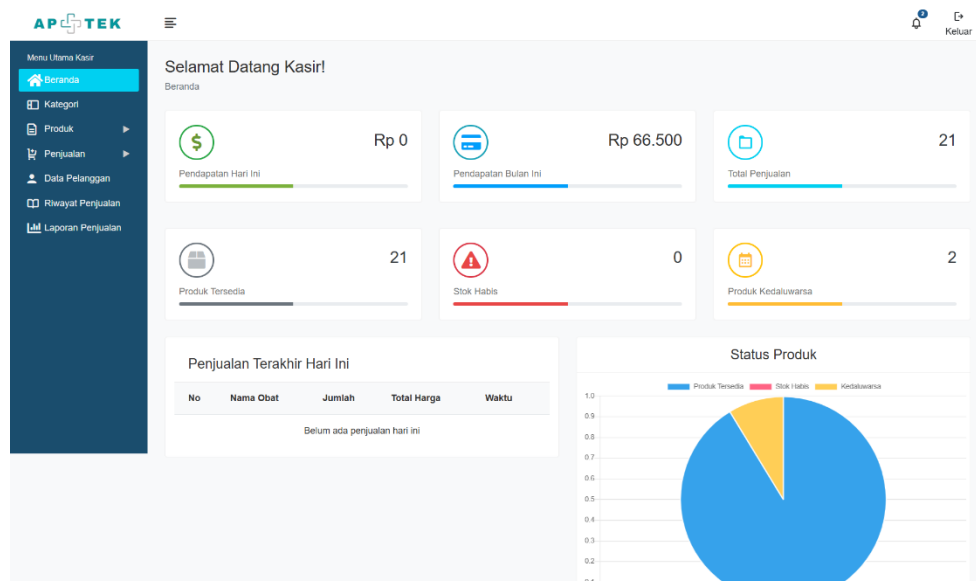
Gambar 4. Beranda
