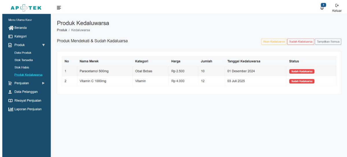
Gambar 8. Produk Kedaluwarsa
