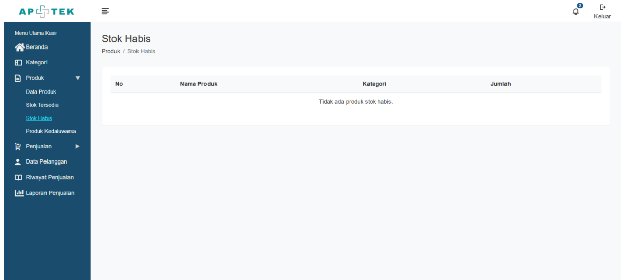
Gambar 7. Stok Habis
